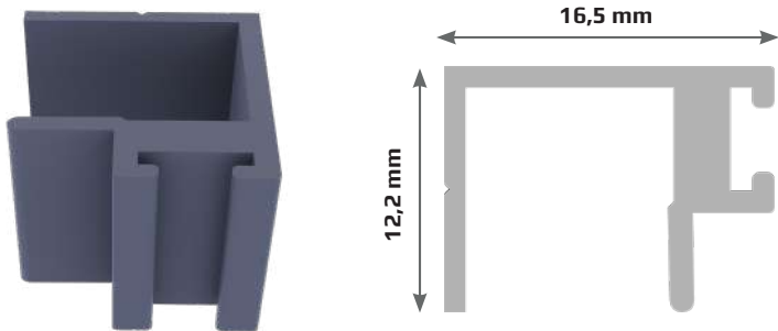
14592 5 Větrací lišta Zugluftdichtung | Draught strip | Tozluk
