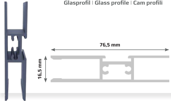
17825 7 Nosný blok Mitnehmerblock | Carrier block | Taşıma bloğu
